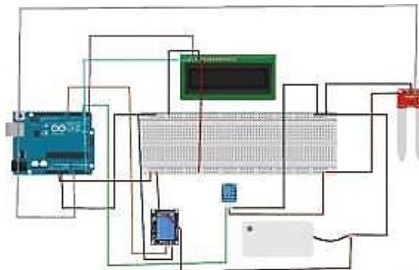
Gambar 4. Rangkaian Skematik
